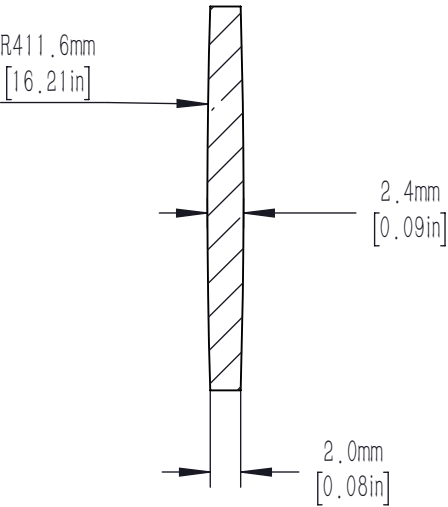
SCETION A-A
